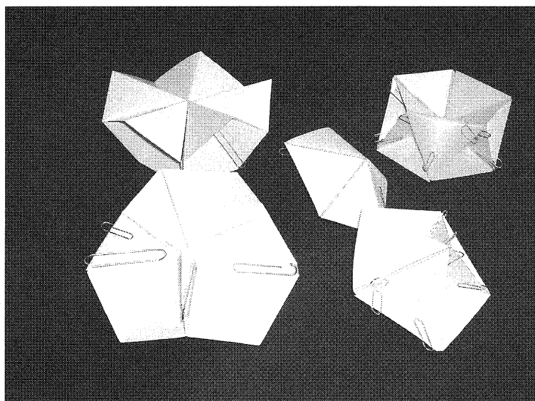
正十二面体と正二十面体のスケルトン模型
