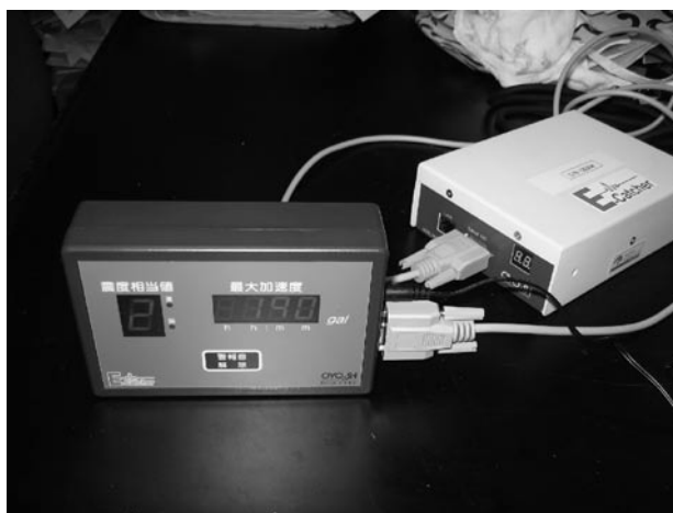
写真1 小型地震計(右)と震度表示装置(左)
